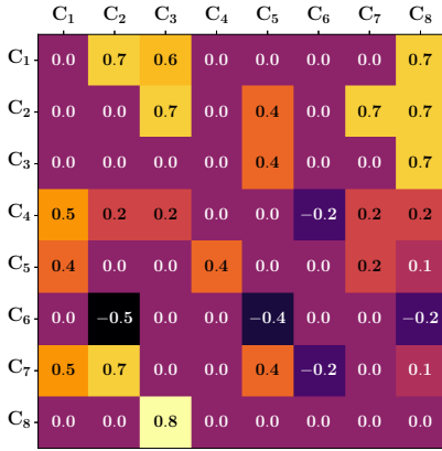
(a) Target edge matrix: E
